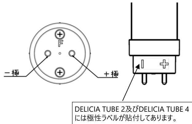
図3：口金の極性に関して
