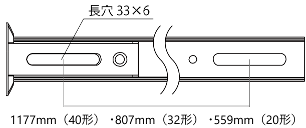
図1：ホルダー推奨取付穴
