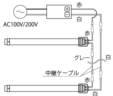
<図9: 2灯配線簡易図>
