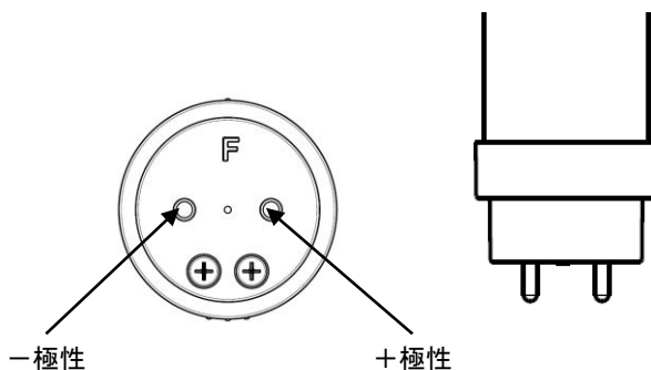
<図3: 口金の極性に関して>
