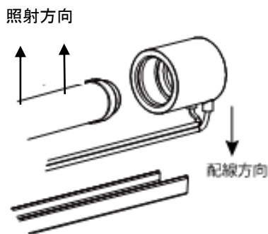
DELICIA TUBE 1 照射方向
