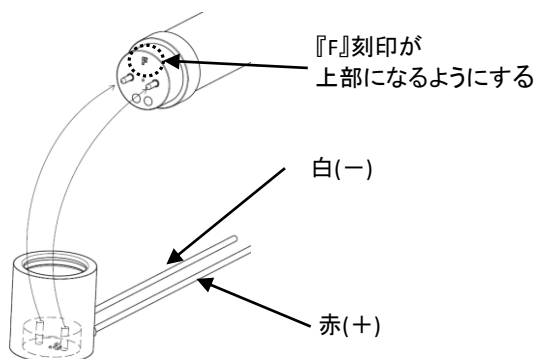
<図2: 嵌め込み向き>
